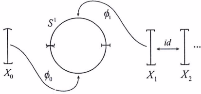
FIG. 1. Limit space (not fundamental)
